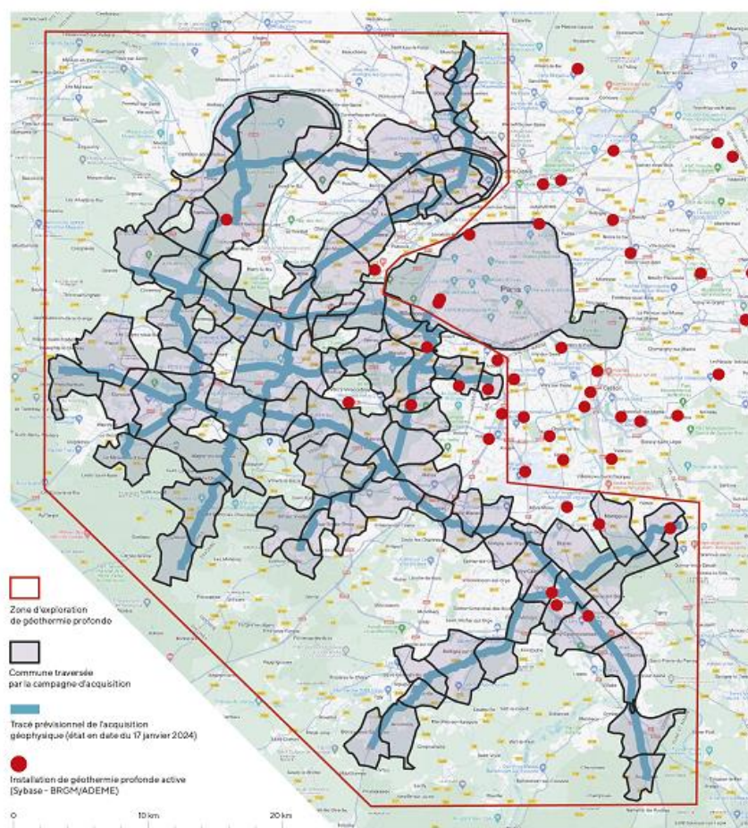
Figure 71 : Exploration du potentiel géothermique en profondeur autour de Paris (BRGM)
